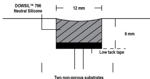
Obr. 2: Mělký spoj
