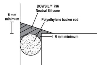
Obr. 3: Koutový spoj
