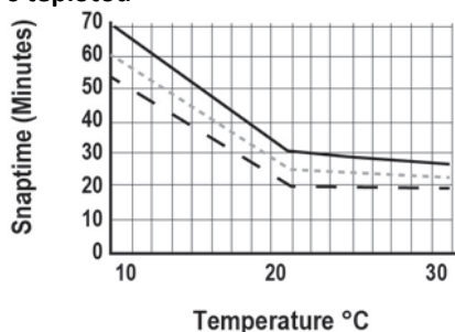
Obr. 2 DOWSIL™ 3362 Tmel na izolační skla – vývoj pracovního času s teplotou
