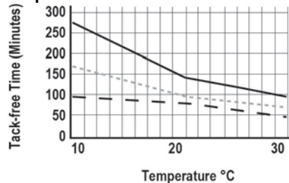
Obr. 3 DOWSIL™ 3362 Tmel na izolační skla – vývoj tvorby slupky s teplotou
